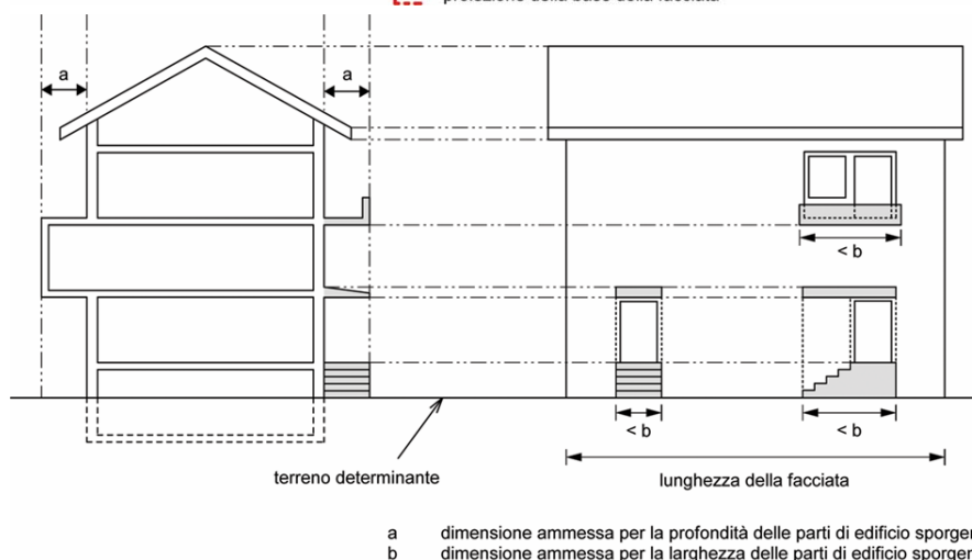
Figura 3.4 Parti di edificio sporgenti (in sezione e in vista laterale)
