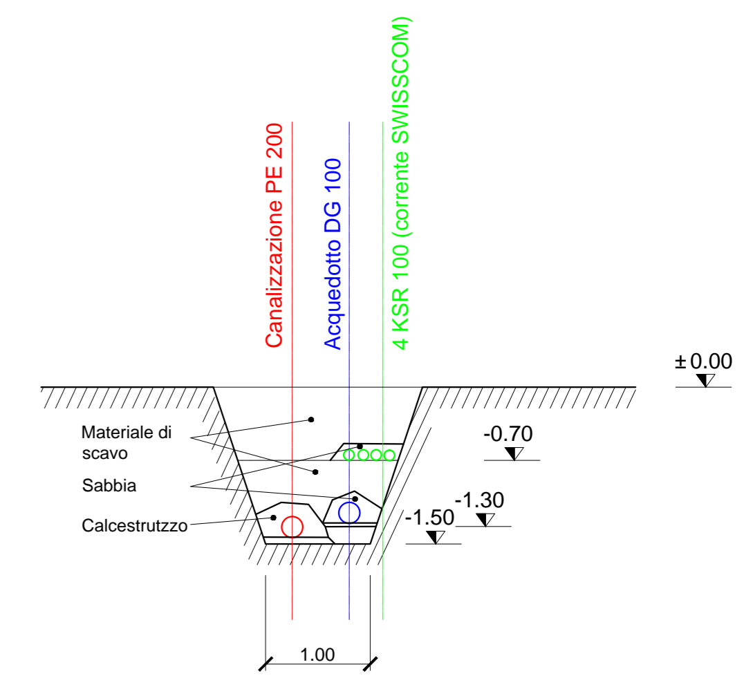
Profilo tipo 1:50
